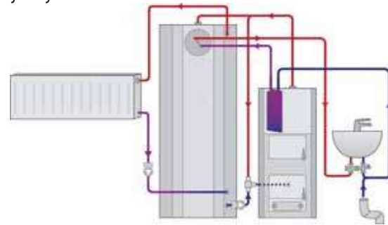
Jäspi Biotriplex energiavaraajan yhteydessä
