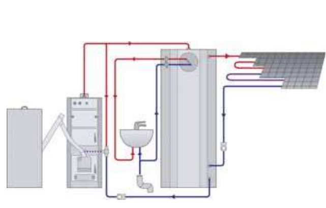
Jäspi Pelletti 25 energiavaraajaan kytkettynä
