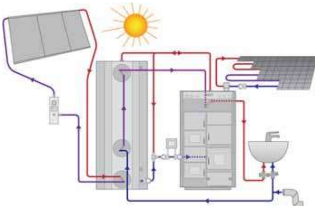
Jäspi Biotriplex energiavaraajan yhteydessä, aurinkopiiriin kytkettynä
