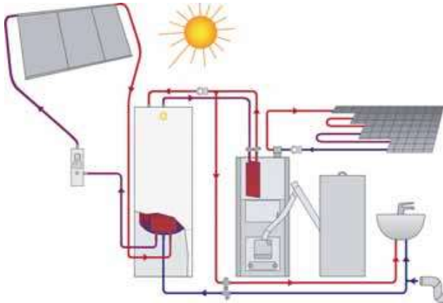
Jäspi Biotriplex energiavaraajan yhteydessä, aurinkopiiriin kytkettynä
