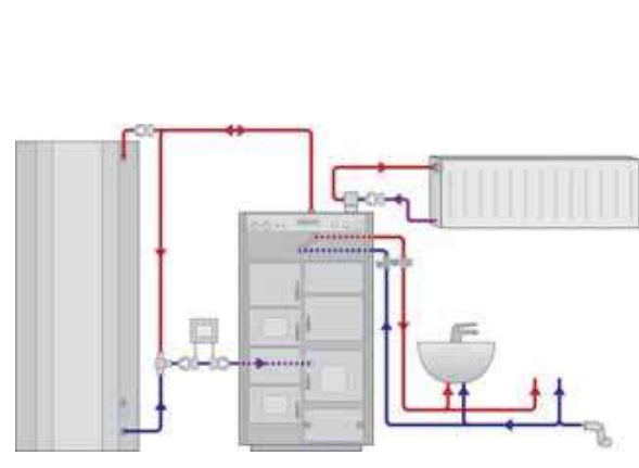
Jäspi Pelletti 25 energiavaraajaan kytkettynä
