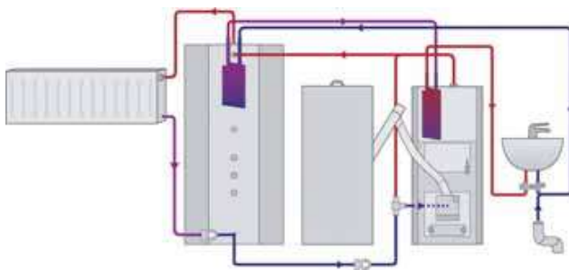
Jäspi Pelletti XL Jäspi Solar Economy PAK:n yhteydessä
